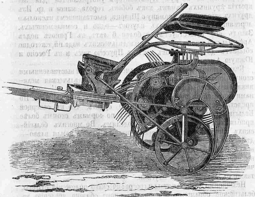
Вращающійся зубчатникъ.
