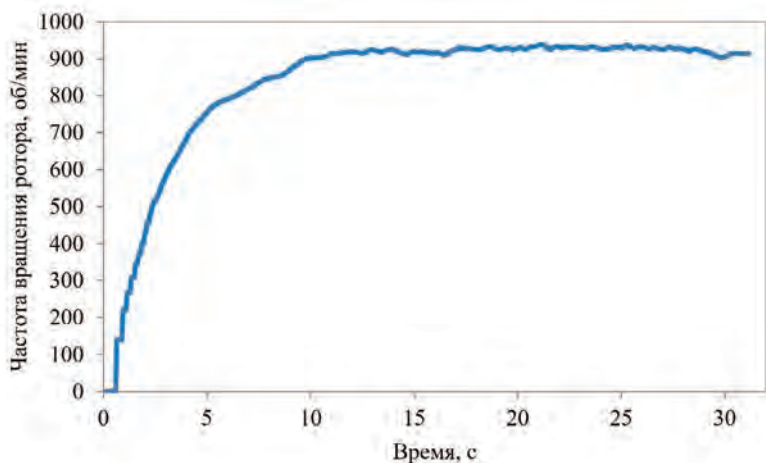
Рисунок 8. Частотно-временная характеристика ротора при d/H = 1/1
