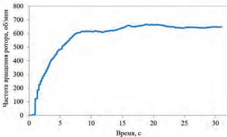
Рисунок 9. Частотно-временная характеристика ротора при d/H = 3/2
