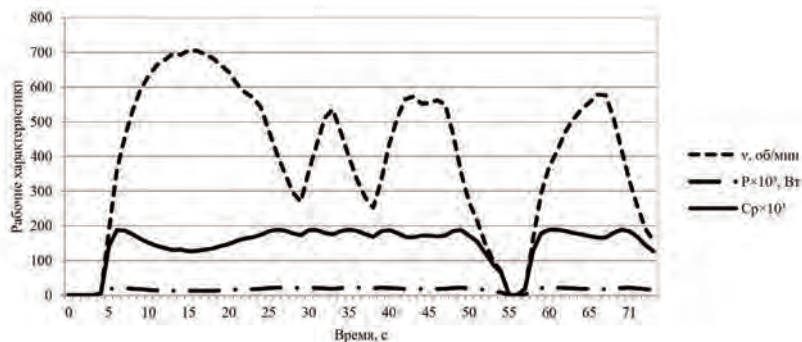
Рисунок 11. Частотно-временная характеристика ротора с соотношением d/H = 3/2 в процессе регулирования
