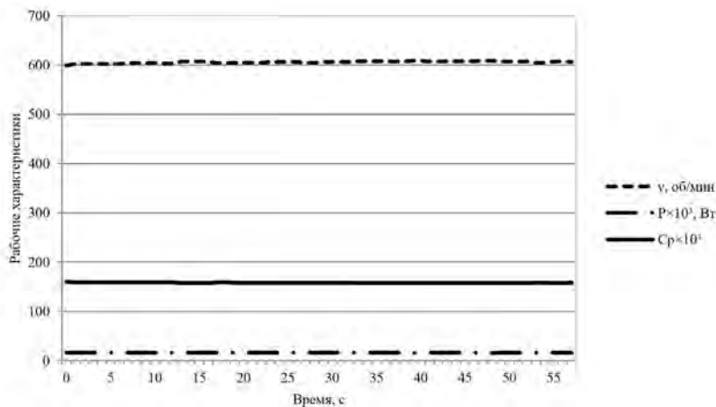
Рисунок 12. Частотно-временная характеристика ротора с соотношением d/H = 3/2 в установившемся процессе
