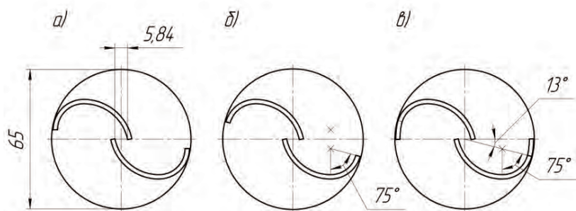
Рисунок 2. Профили ротора: а) 1 вариант; б) 2 вариант; в) 3 вариант
