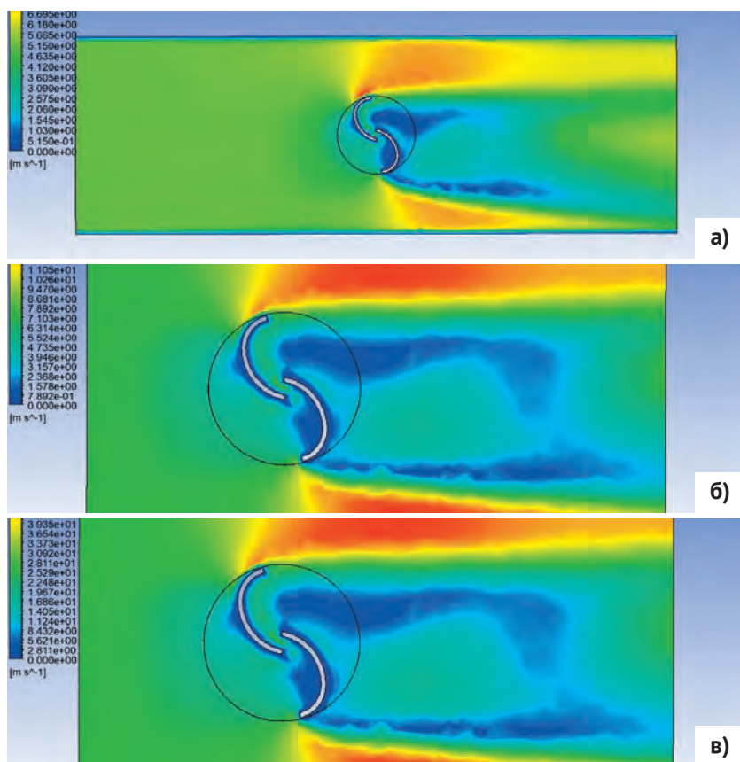
Рисунок 6. Скоростные поля: а) при v = 5 м/с; б) при v = 10 м/с; в) при v = 25 м/с
