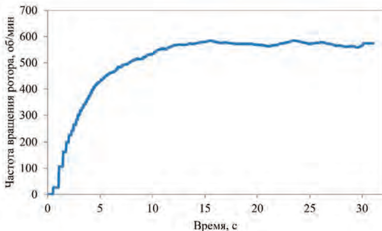
Рисунок 10. Частотно-временная характеристика ротора при d/H = 2/1
