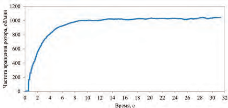
Рисунок 7. Частотно-временная характеристика ротора при d/H = 2/3
